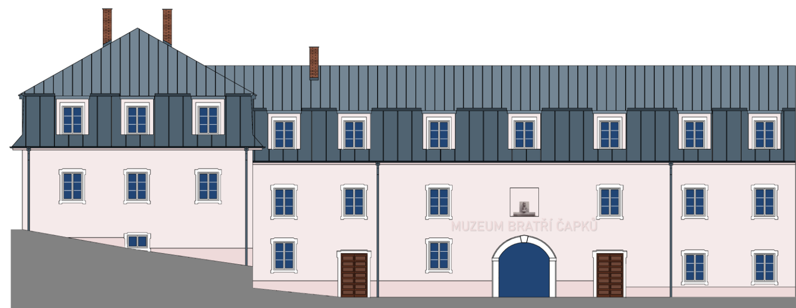
SEVERNÍ POHLED
