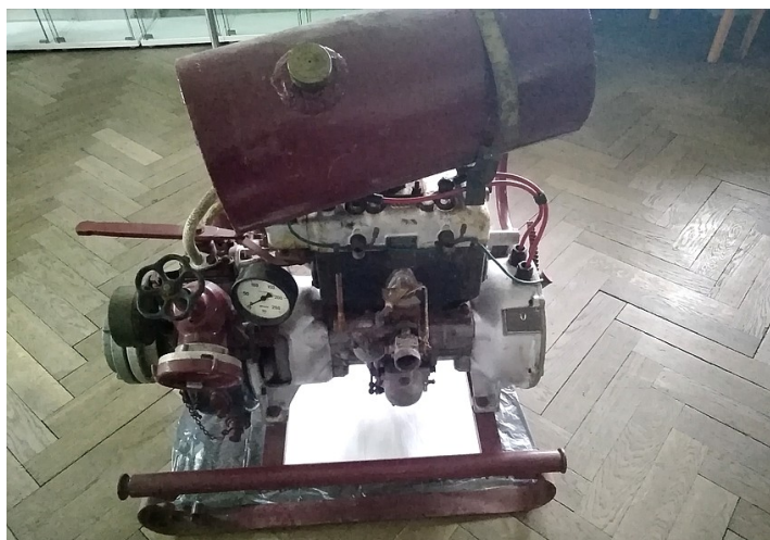
Exponát č. 33: Přenosná stříkačka PS-8 DKW.
