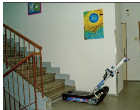
Nový schodolez
